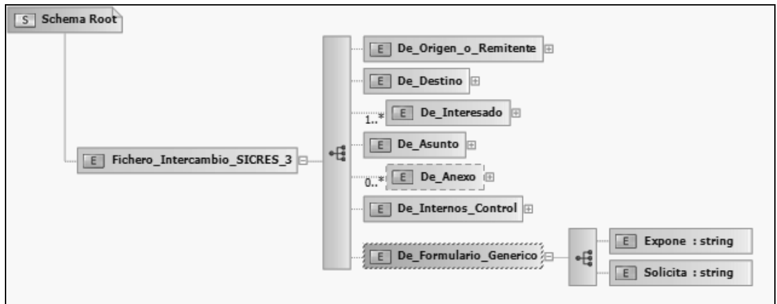
Figura 19. Esquema XML: Mensaje de datos de intercambio - Detalle de Formulario Genérico.
