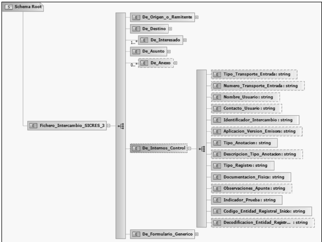
Figura 18. Esquema XML: Mensaje de datos de intercambio - Detalle de Internos y Control.
